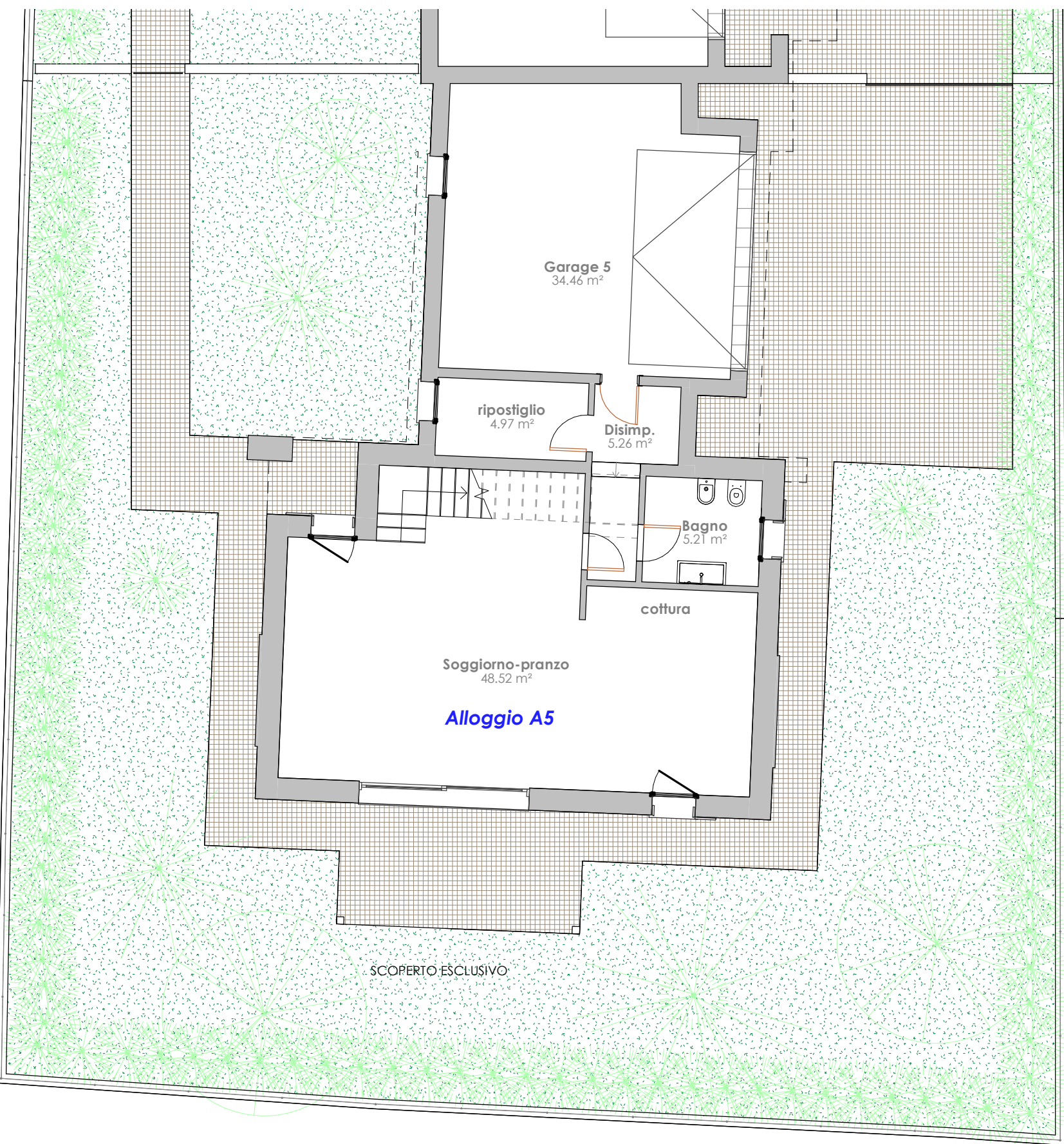
PIANTA PIANO TERRA sc 1:100
