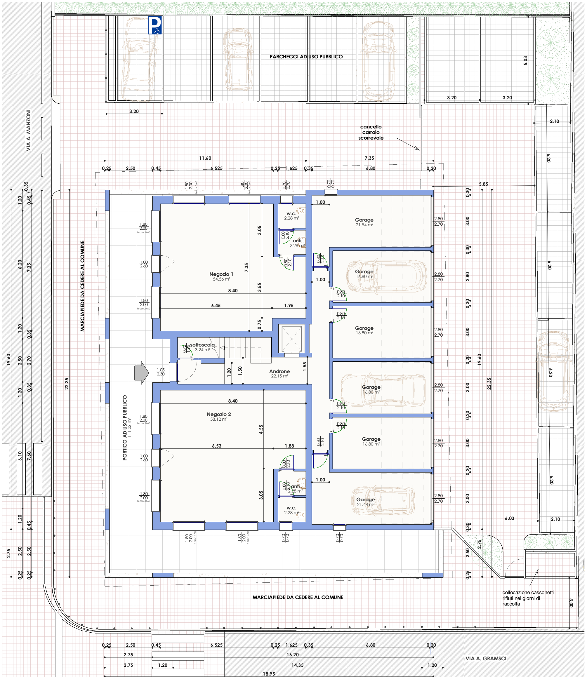
PLANIMETRIA CON PIANTA PIANO TERRA
